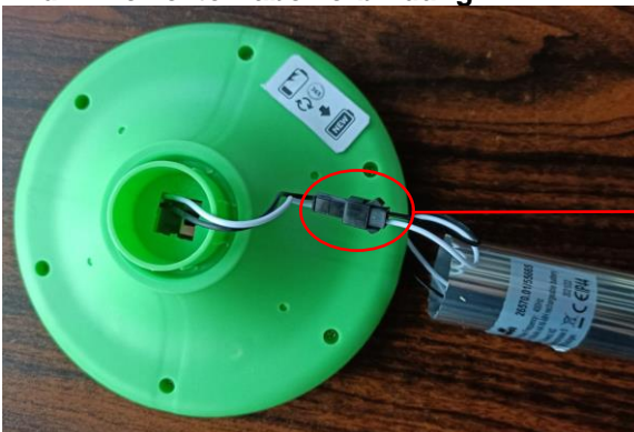
Bild 2: Korrekte Kabelverbindung
